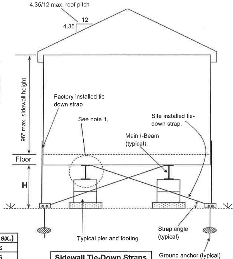
Sidewall Tie-Down Straps
